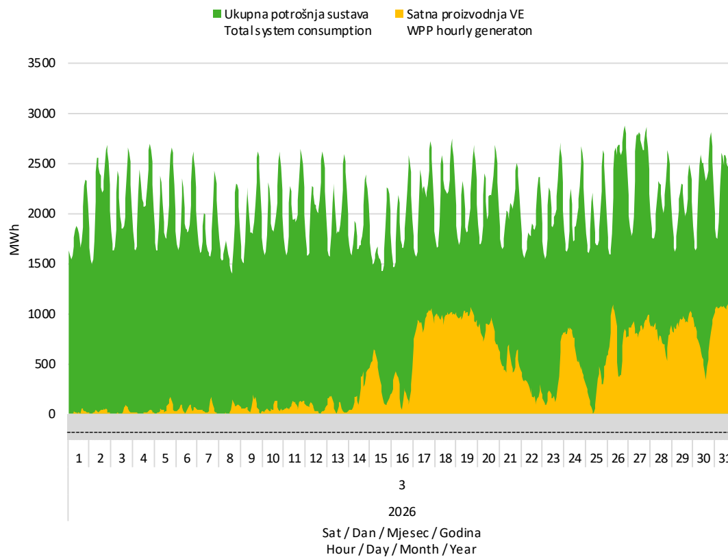
Slika 7 Usporedba satnog dijagrama opterećenja sustava i proizvodnje vjetroelektrana u ožujku 2026. godine
