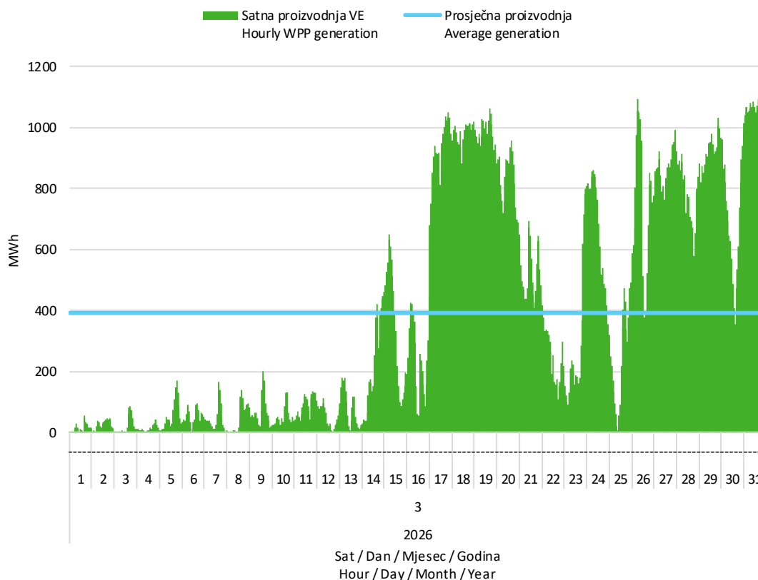
Slika 2 Satna proizvodnja svih vjetroelektrana u ožujku 2026. godine
