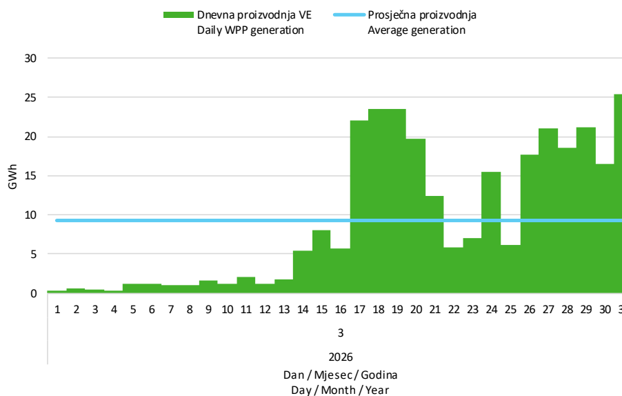
Slika 5 Dnevna proizvodnja svih vjetroelektrana u ožujku 2026. godine
