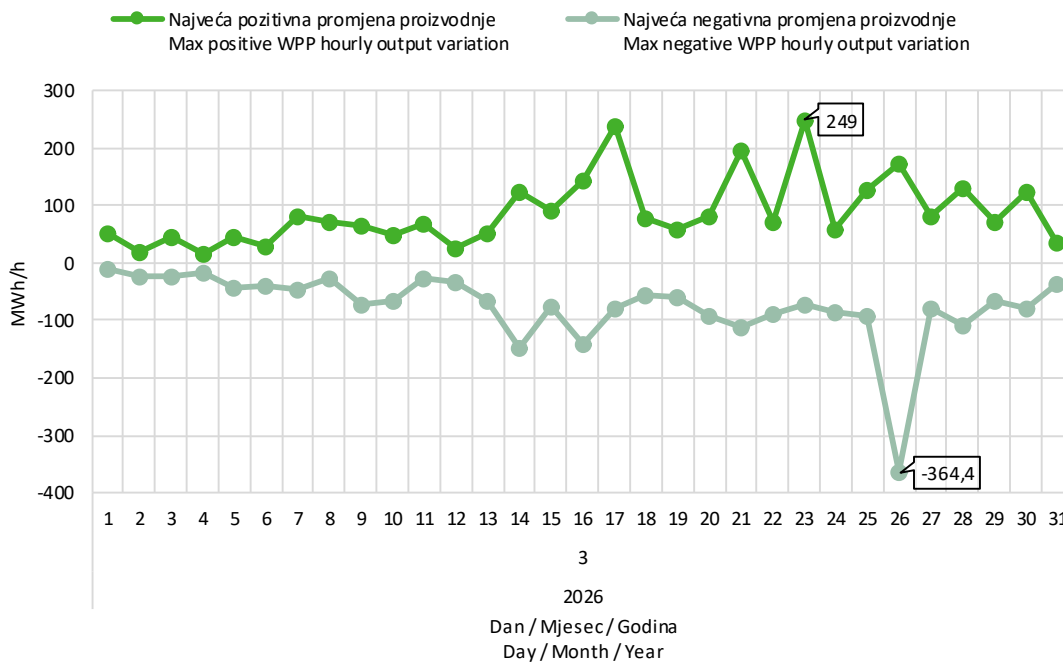
Slika 9 Maksimalna pozitivna i maksimalna negativna promjena satne proizvodnje VE u ožujku 2026. godine
