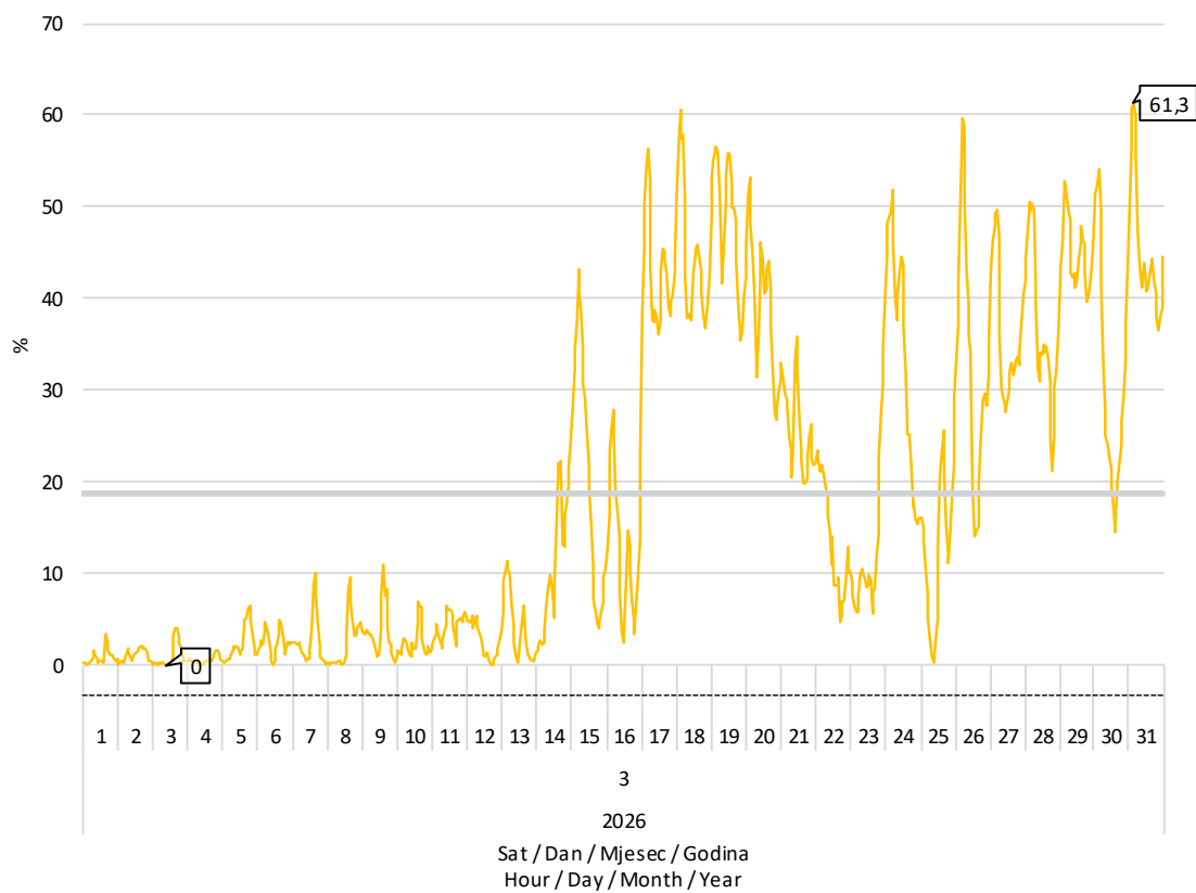
Slika 8 Udio proizvodnje vjetroelektrana u pokrivanju satnog opterećenja elektroenergetskog sustava u ožujku 2026. godine
