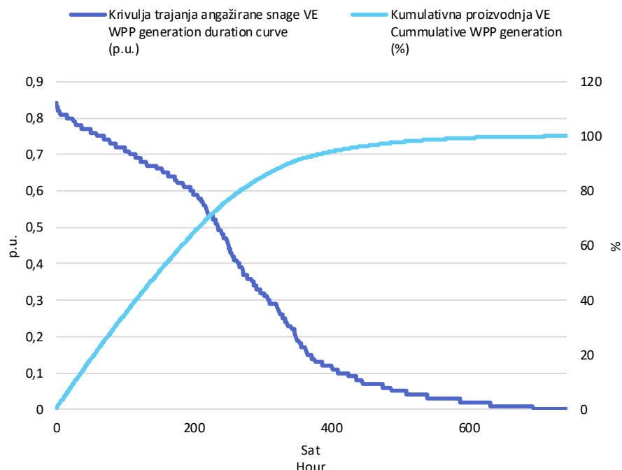
Slika 3 Krivulja trajanja angažirane snage svih VE i kumulativna proizvodnja VE u ožujku 2026. godine u jediničnim vrijednostima
