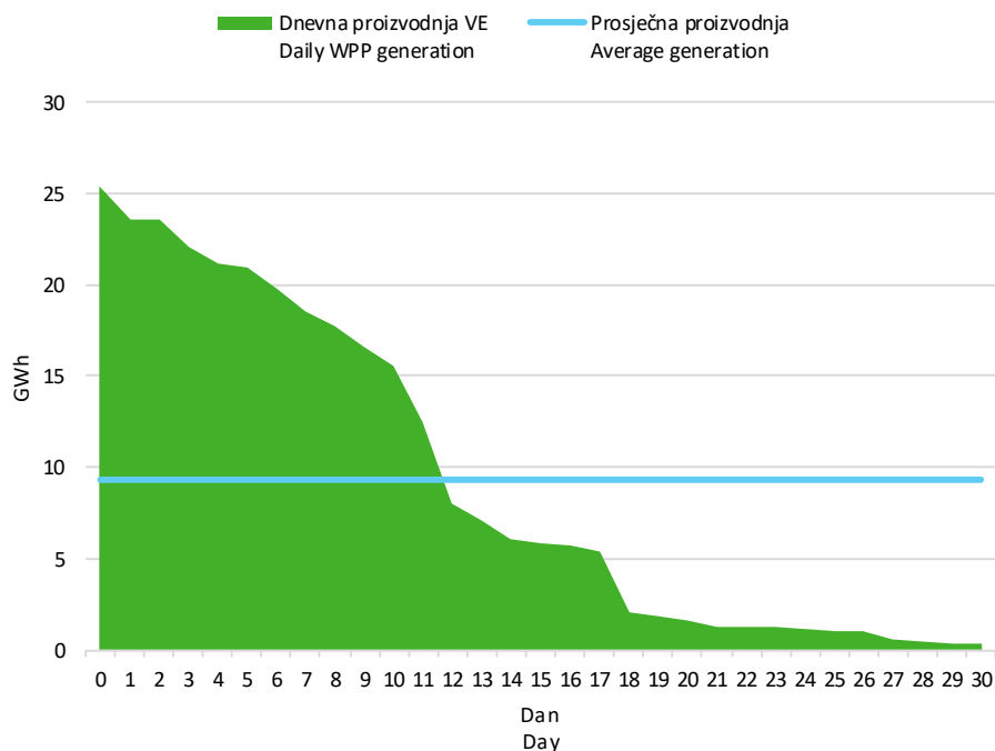
Slika 6 Krivulja trajanja dnevne proizvodnje vjetroelektrana u ožujku 2026. godine
